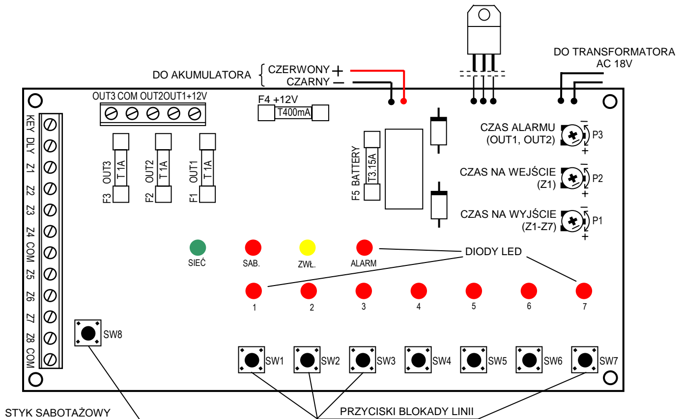
Rysunek 1. Widok płytki centrali w wykonaniu CA8MX V1.1
